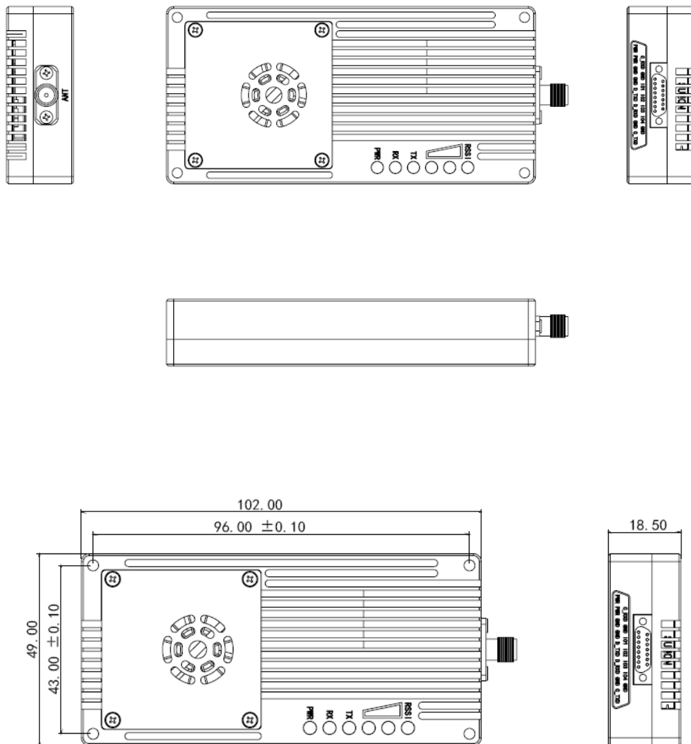
T900-40-SMA 尺寸示意图
